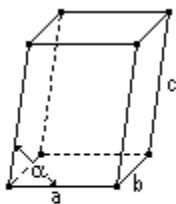
MONOCLINIC
